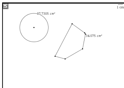
圓形或多邊形的面積
