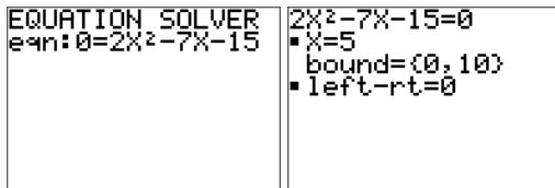
Numerieke oplosser
