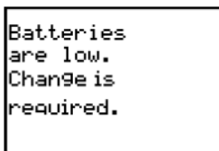
Bericht B
