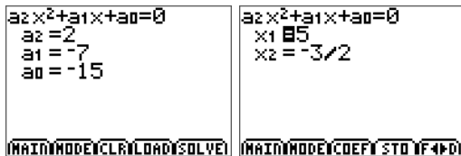
Veeltermoplosser
