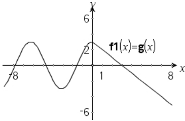
g(x) 繪圖結果
