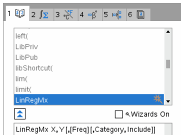
LinRegMx function in a CAS handheld
