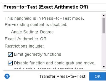
Eksakt aritmetik-OS
